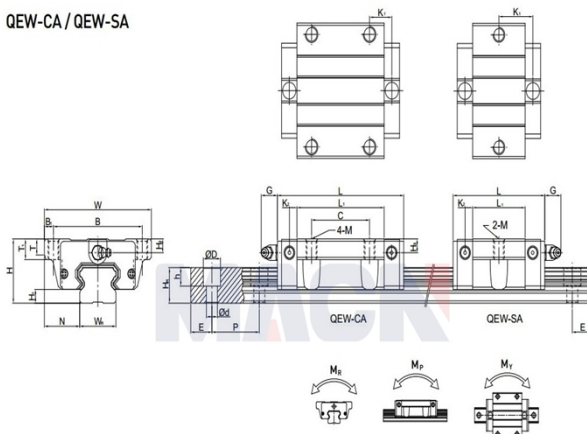
下锁式滑轨
